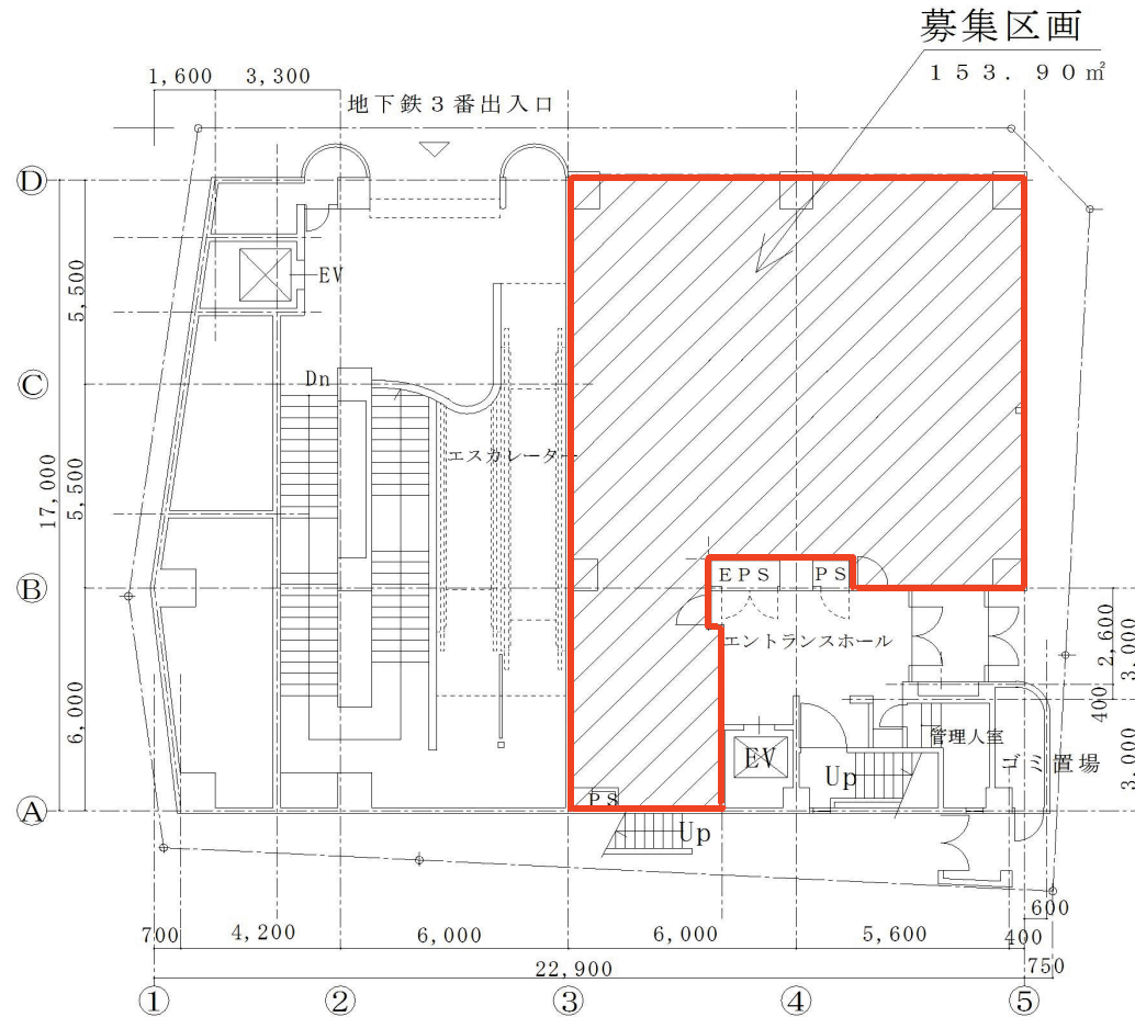
1階 平面図
