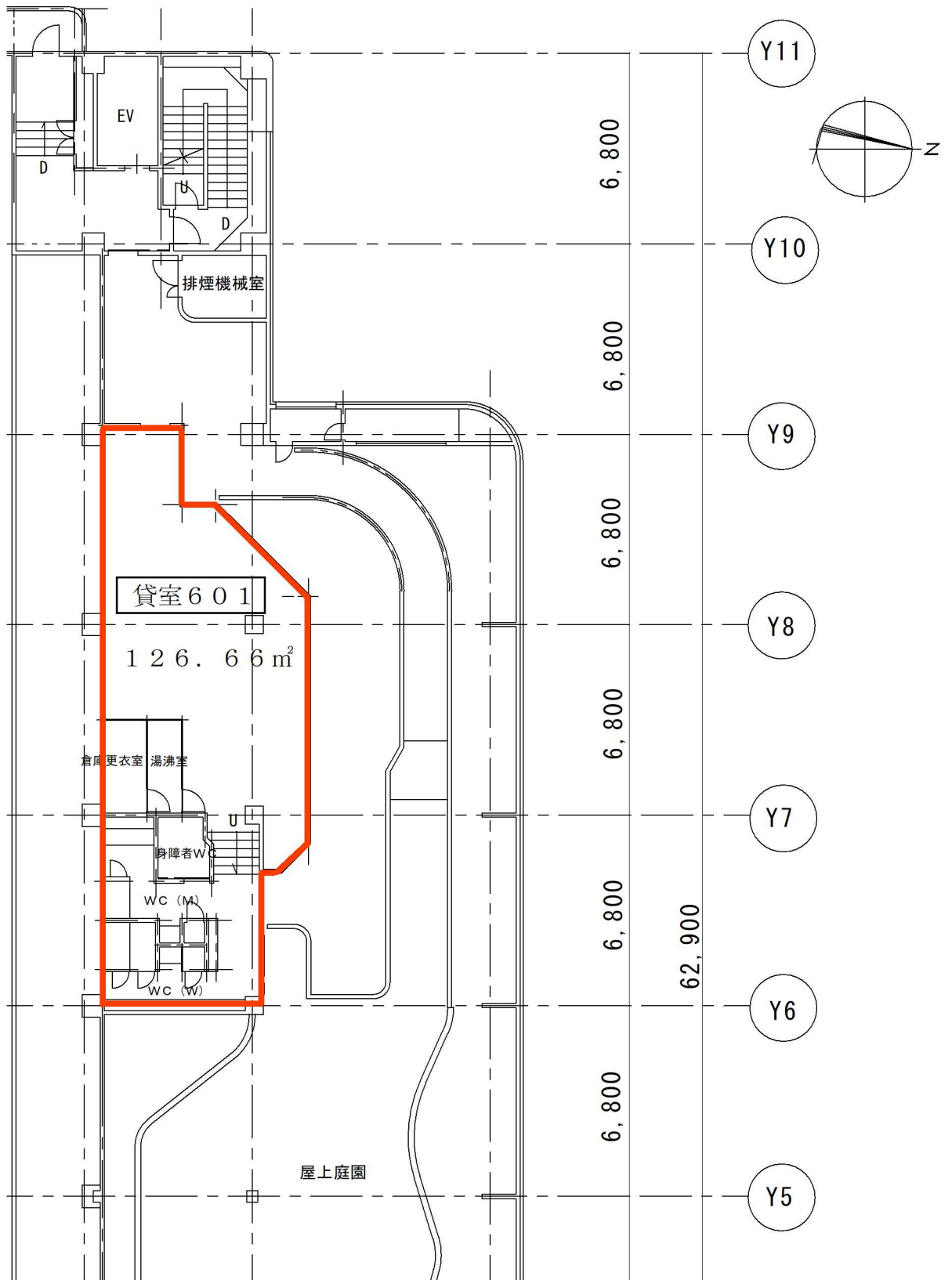
6 階平面図
