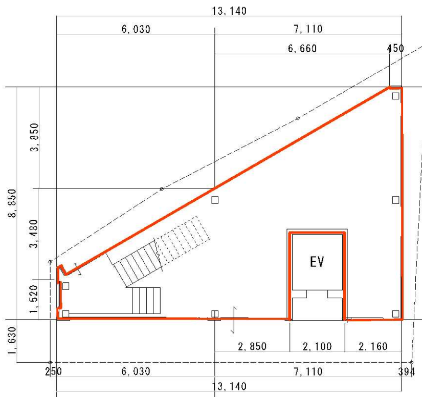
1階平面図
