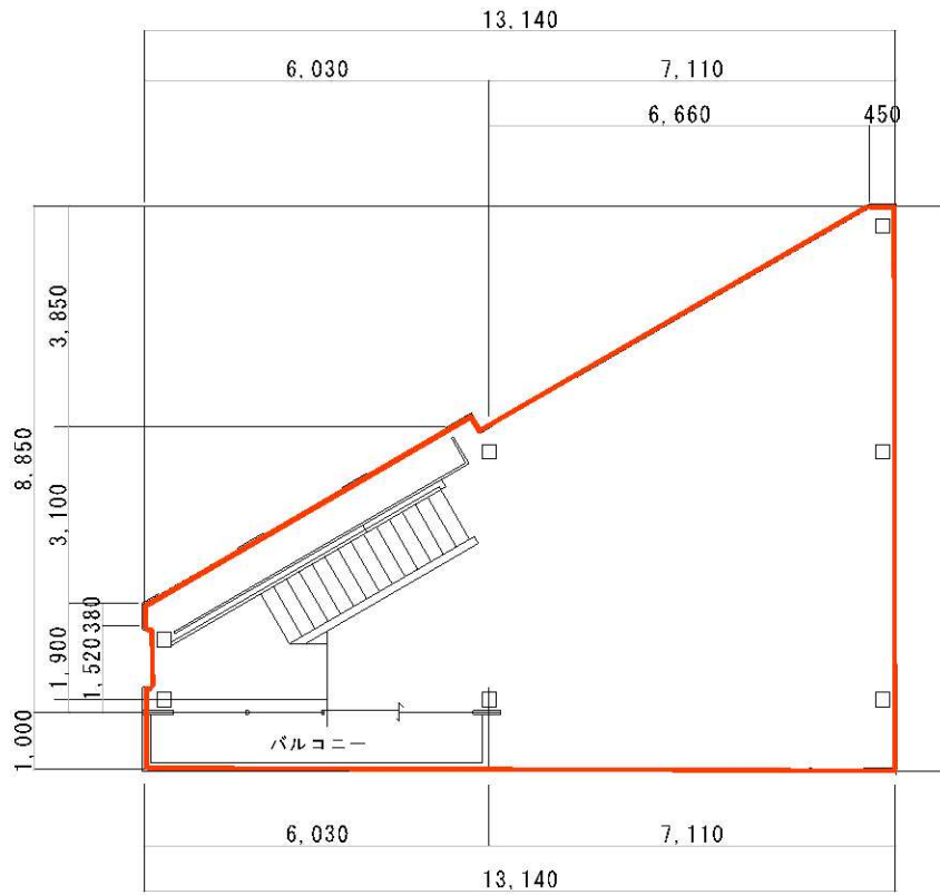
2階平面図
